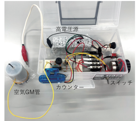
図 3：簡易型空気 GM 管の完成写真
